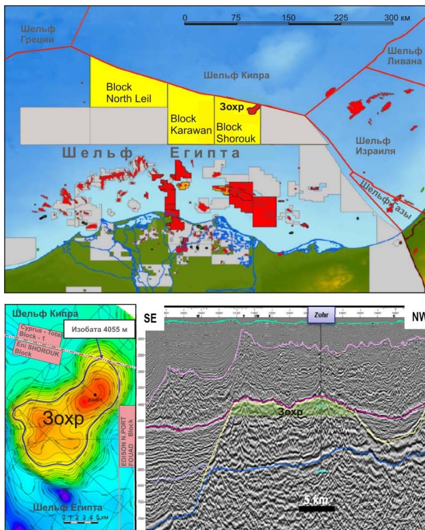
Рис. 5. Расположение гигантского газового месторождения Зохран шельфе Средиземного моря, его план и сейсмический разрез
